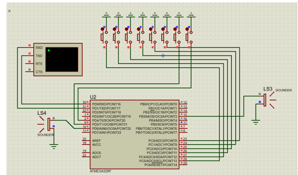
Figura 24. Simulación en Proteus del sistema de piano electrónico. Se observa la activación de los pulsadores, la generación de tonos en el buzzer y la respuesta del microcontrolador ATmega328P configurado con interrupciones PCINT . Fuente: elaboración propia.
