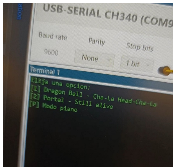
Figura 13. Interfaz de comunicación serial (USART) mostrando el menú de control del módulo Piano . Desde la terminal, el usuario puede seleccionar entre el modo manual por pulsadores o la reproducción automática de melodías predefinidas. Fuente: elaboración propia.
