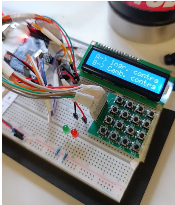
Figura 14. Montaje del circuito correspondiente al sistema de cerradura electrónica. Se observa la conexión del teclado matricial 4x4, la pantalla LCD 16x2 con interfaz I2C, los indicadores luminosos (LED rojo y verde), el buzzer de alarma y el microcontrolador ATmega328P. Fuente: elaboración propia.
