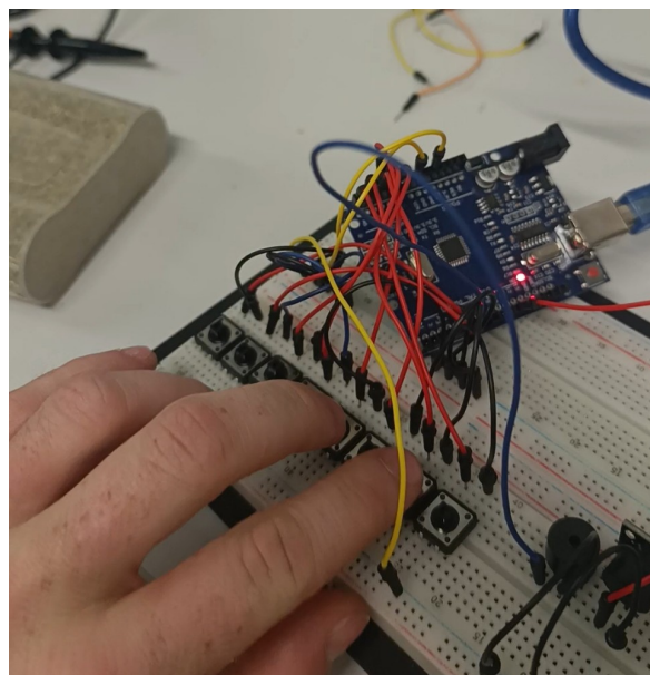
Figura 12. Montaje del circuito correspondiente al módulo Piano , compuesto por el microcontrolador ATmega328P, el buzzer piezoeléctrico, los pulsadores de entrada y los componentes de conexión. Fuente: elaboración propia.
