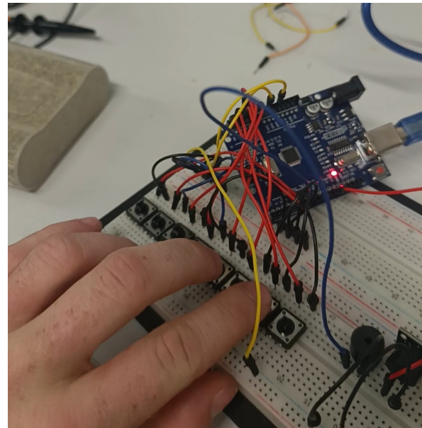
Figura 25. Montaje del circuito correspondiente al módulo Piano , compuesto por el microcontrolador ATmega328P, el buzzer piezoeléctrico, los pulsadores de entrada y los componentes de conexión. Fuente: elaboración propia.
