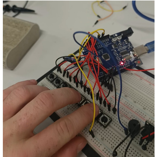
Figura 12. Montaje del circuito correspondiente al módulo Piano , compuesto por el microcontrolador ATmega328P, el buzzer piezoeléctrico, los pulsadores de entrada y los componentes de conexión. Fuente: elaboración propia.
