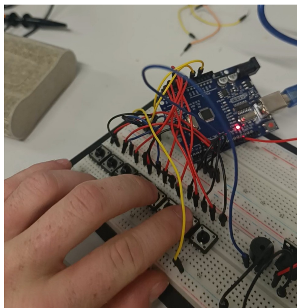
Figura 17. Montaje del circuito correspondiente al módulo Piano , compuesto por el microcontrolador ATmega328P, el buzzer piezoeléctrico, los pulsadores de entrada y los componentes de conexión. Fuente: elaboración propia.
