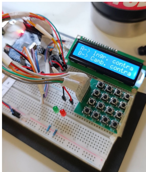
Figura 20. Montaje del circuito correspondiente al sistema de cerradura electrónica. Se observa la conexión del teclado matricial 4x4, la pantalla LCD 16x2 con interfaz I2C, los indicadores luminosos (LED rojo y verde), el buzzer de alarma y el microcontrolador ATmega328P. Fuente: elaboración propia.
