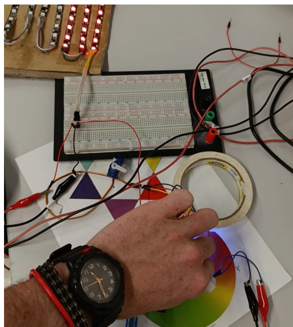
Figura 14. Identificación de color efectiva. Fuente: elaboración propia
