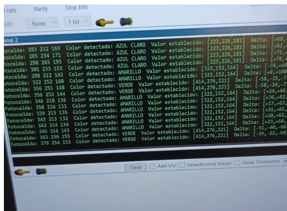
Figura 15. Identificación de color efectiva mediante comunicación serial a través de la terminal. Se observa la lectura del valor ADC, el color detectado, el valor establecido y la desviación del mismo. Fuente: elaboración propia.
