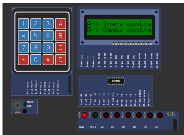
Figura 19. Simulación en PicSimLab del sistema de cerradura electrónica. Se observan los periféricos principales: teclado matricial, pantalla LCD, LEDs indicadores y buzzer, así como la correcta ejecución de las rutinas de interfaz y control de estado. Fuente: elaboración propia.
