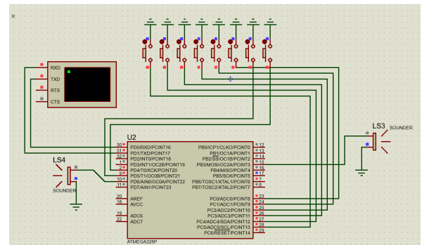
Figura 21. Simulación en Proteus del sistema de piano electrónico. Se observa la activación de los pulsadores, la generación de tonos en el buzzer y la respuesta del microcontrolador ATmega328P configurado con interrupciones PCINT. Fuente: elaboración propia.
