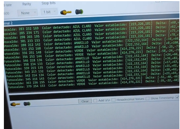
Figura 20. Identificación de color efectiva mediante comunicación serial a través de la terminal. Se observa la lectura del valor ADC, el color detectado, el valor establecido y la desviación del mismo. Fuente: elaboración propia.
