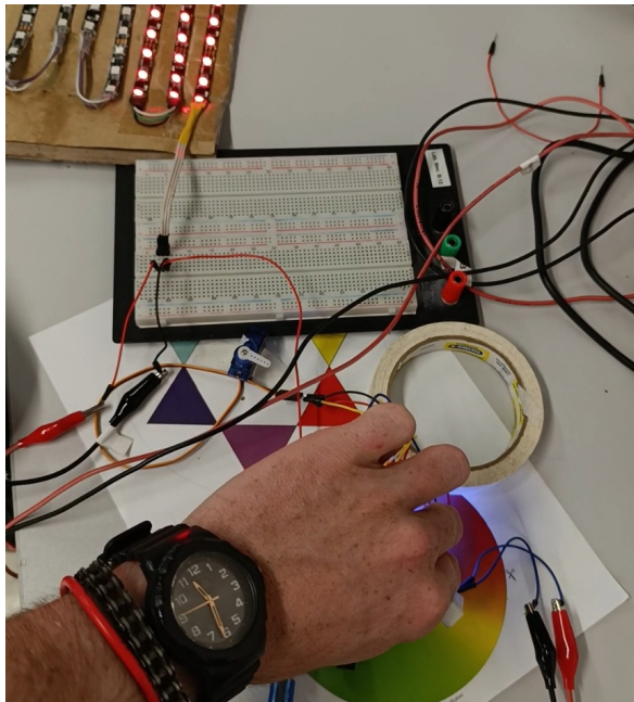
Figura 19. Identificación de color efectiva. Fuente: elaboración propia.
