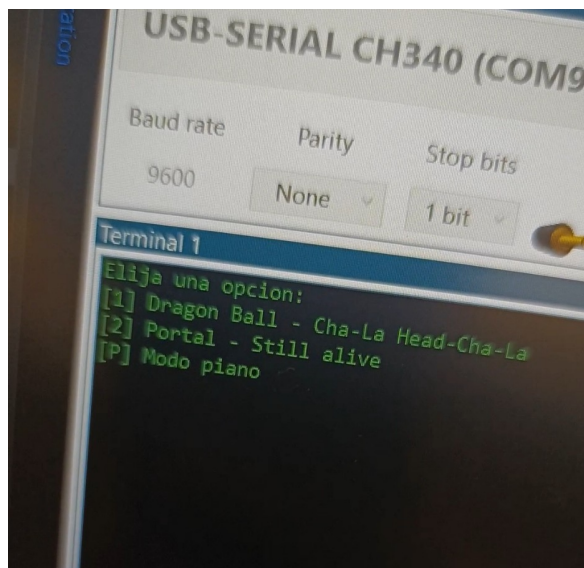
Figura 23. Interfaz de comunicación serial ( USART ) mostrando el menú de control del módulo Piano . Desde la terminal, el usuario puede seleccionar entre el modo manual por pulsadores o la reproducción automática de melodías predefinidas. Fuente: elaboración propia.
