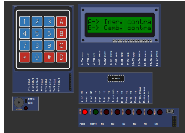
Figura 16. Simulación en PicSimLab del sistema de cerradura electrónica. Se observan los periféricos principales: teclado matricial, pantalla LCD, LEDs indicadores y buzzer, así como la correcta ejecución de las rutinas de interfaz y control de estado. Fuente: elaboración propia.
