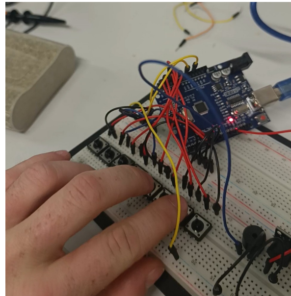
Figura 14. Montaje del circuito correspondiente al módulo Piano , compuesto por el microcontrolador ATmega328P, el buzzer piezoeléctrico, los pulsadores de entrada y los componentes de conexión. Fuente: elaboración propia.
