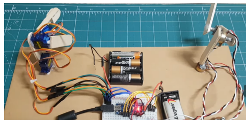
Figura 18: Controlador espejo con potenciómetros TechZone (2021)
