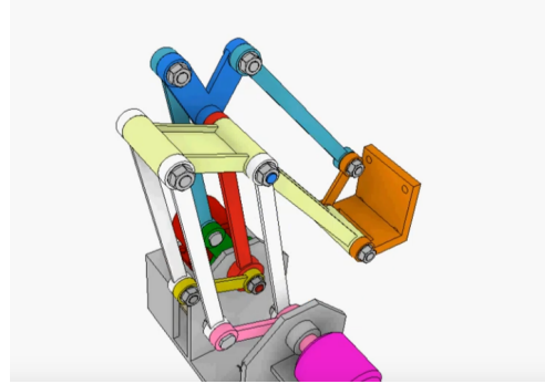
Figura 12: Sistema de eslabones con mayor libertad Thang010146 (2021).
