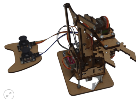
Figura 10: Control por joystick Robodacta (2022a)
