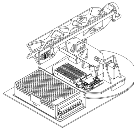
Figura 12: Diseño con eslabones y servomotores mg996r (Fuente: elaboración propia)
