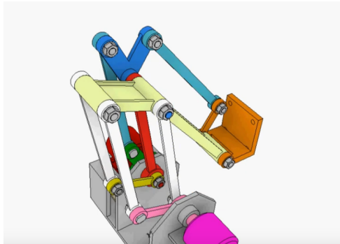
Figura 6: Sistema de eslabones con mayor libertad Thang010146 (2021).
