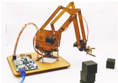
Figura 7: Modelo en MDF Robodacta (2022b).
