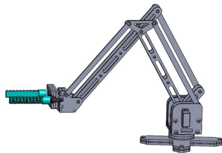
Figura 5: Sistema de eslabones GrabCAD (2021d).
