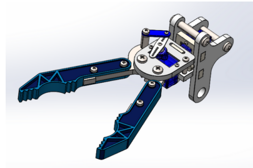
Figura 9: Manipulador por garra y servomotor GrabCAD (2021c).
