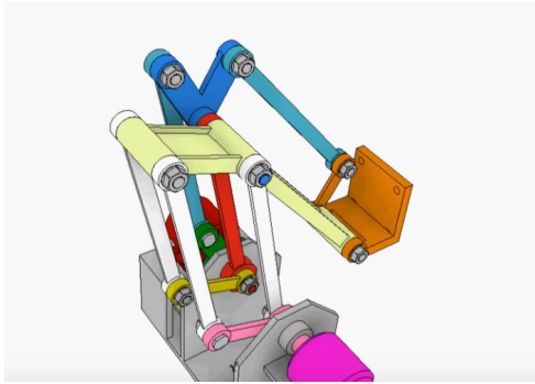
Figura 11: Sistema de eslabones con mayor libertad Thang010146 (2021).
