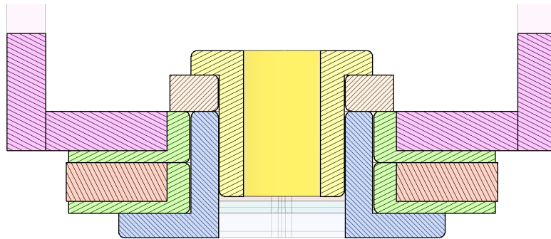
Figura 5: Corte transversal perno — versión mejorada. Fuente: elaboración propia
