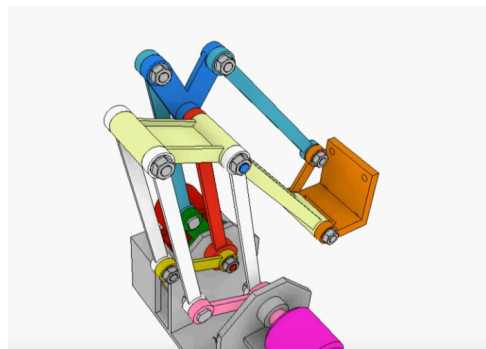
Figura 24: Sistema de eslabones con mayor libertad Thang010146 (2021).
