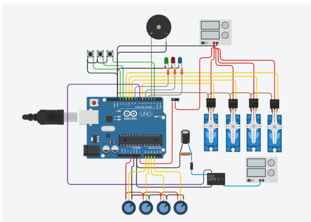
Figura 9: Diagrama de conexiones eléctricas. Fuente: elaboración propia
