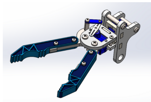
Figura 10: Manipulador por garra y servomotor ?.
