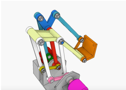
Figura 12: Sistema de eslabones con mayor libertad ?.
