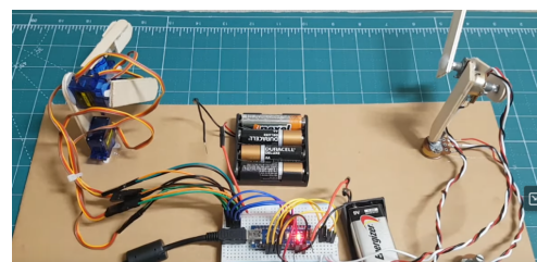
Figura 15: Controlador espejo con potenciómetros ?
