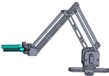
Figura 15: Sistema de eslabones GrabCAD (2021d).
