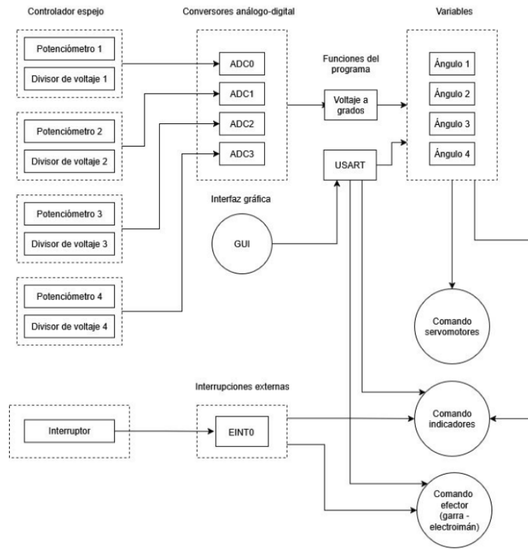
Figura 11: Diagrama de flujo del código en C. Fuente: elaboración propia
