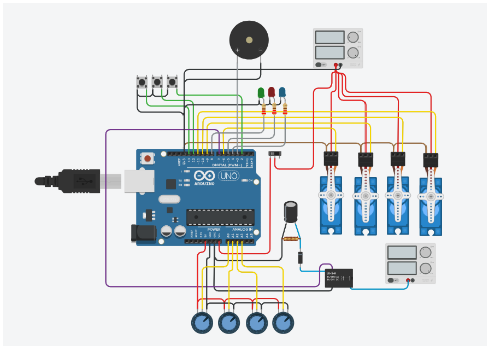
Figura 10: Diagrama de conexiones eléctricas. Fuente: elaboración propia
