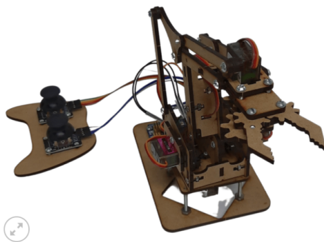
Figura 20: Control por joystick Robodacta (2022a)
