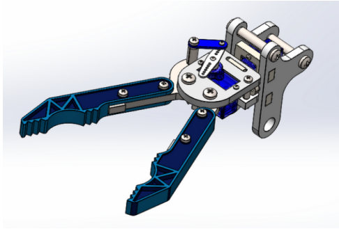
Figura 14: Manipulador por garra y servomotor GrabCAD (2021c).
