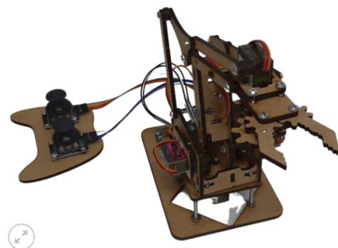
Figura 11: Control por joystick Robodacta (2022a)
