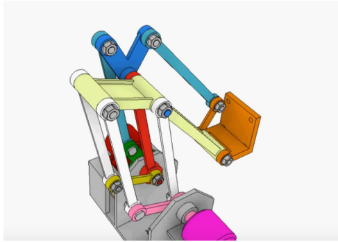
Figura 7: Sistema de eslabones con mayor libertad Thang010146 (2021).
