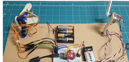
Figura 10: Controlador espejo con potenciómetros TechZone (2021)
