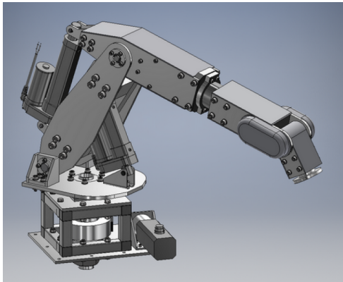
Figura 3: Modelo con actuadores lineales GrabCAD (2021a).
