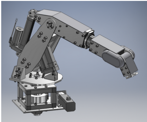
Figura 2: Modelo con actuadores lineales [Gra21a].
