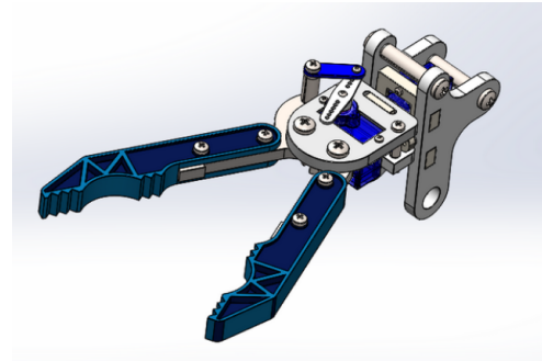
Figura 4: Manipulador por garra y servomotor [Gra21c].
