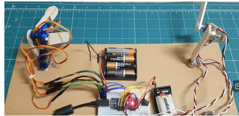
Figura 9: Controlador espejo con potenciómetros [Tec21]
