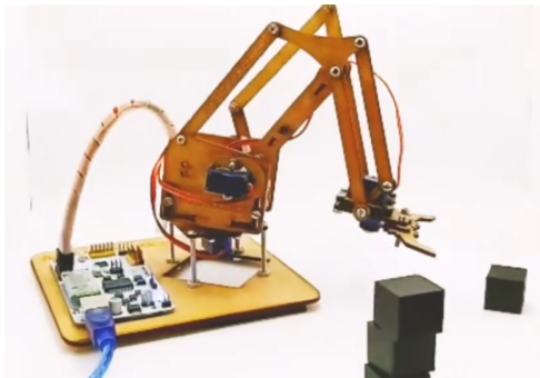
Figura 7: Modelo en MDF [Rob22b].
