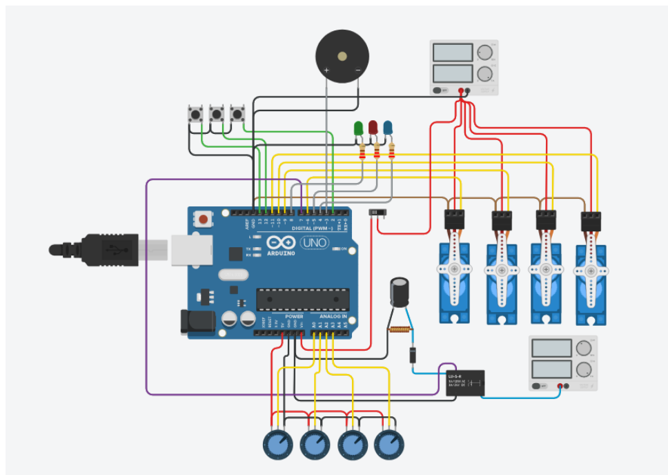
Figura 17: Diagrama de conexiones eléctricas. Fuente: elaboración propia
