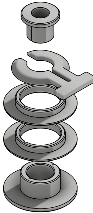
Figura 7: Despiece de articulación desmontable. Fuente: elaboración propia
