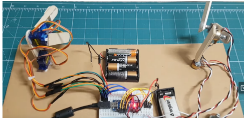
Figura 26: Controlador espejo con potenciómetros TechZone (2021)
