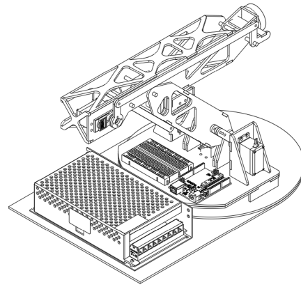
Figura 23: Diseño con eslabones y servomotores mg996r (Fuente: elaboración propia)
