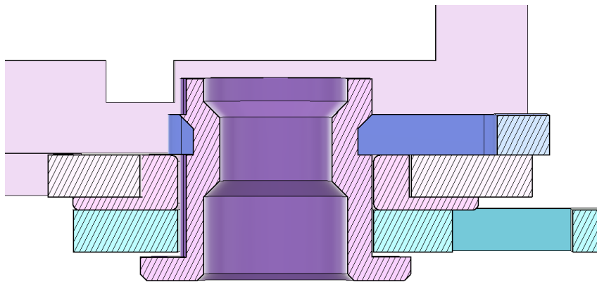
Figura 4: Sistema de articulación desmontable. Fuente: elaboración propia
