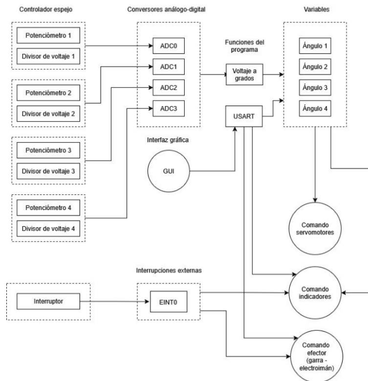
Figura 9: Diagrama de flujo del código en C. Fuente: elaboración propia
