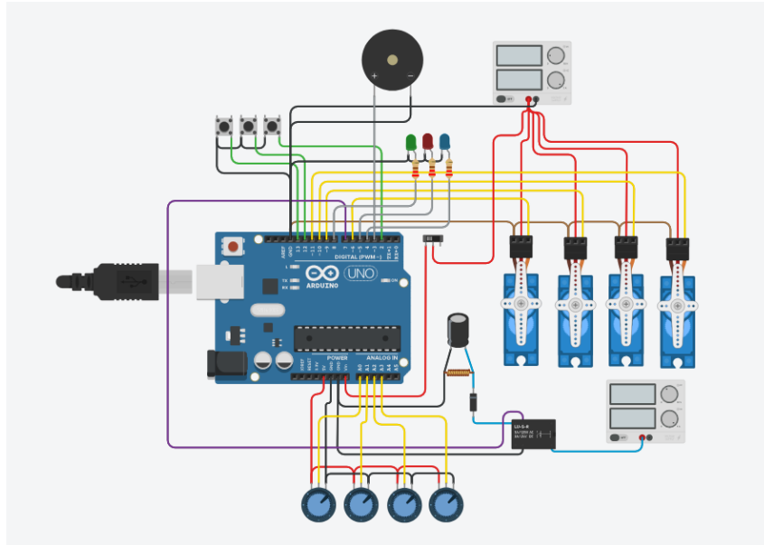
Figura 10: Diagrama de conexiones eléctricas. Fuente: elaboración propia
