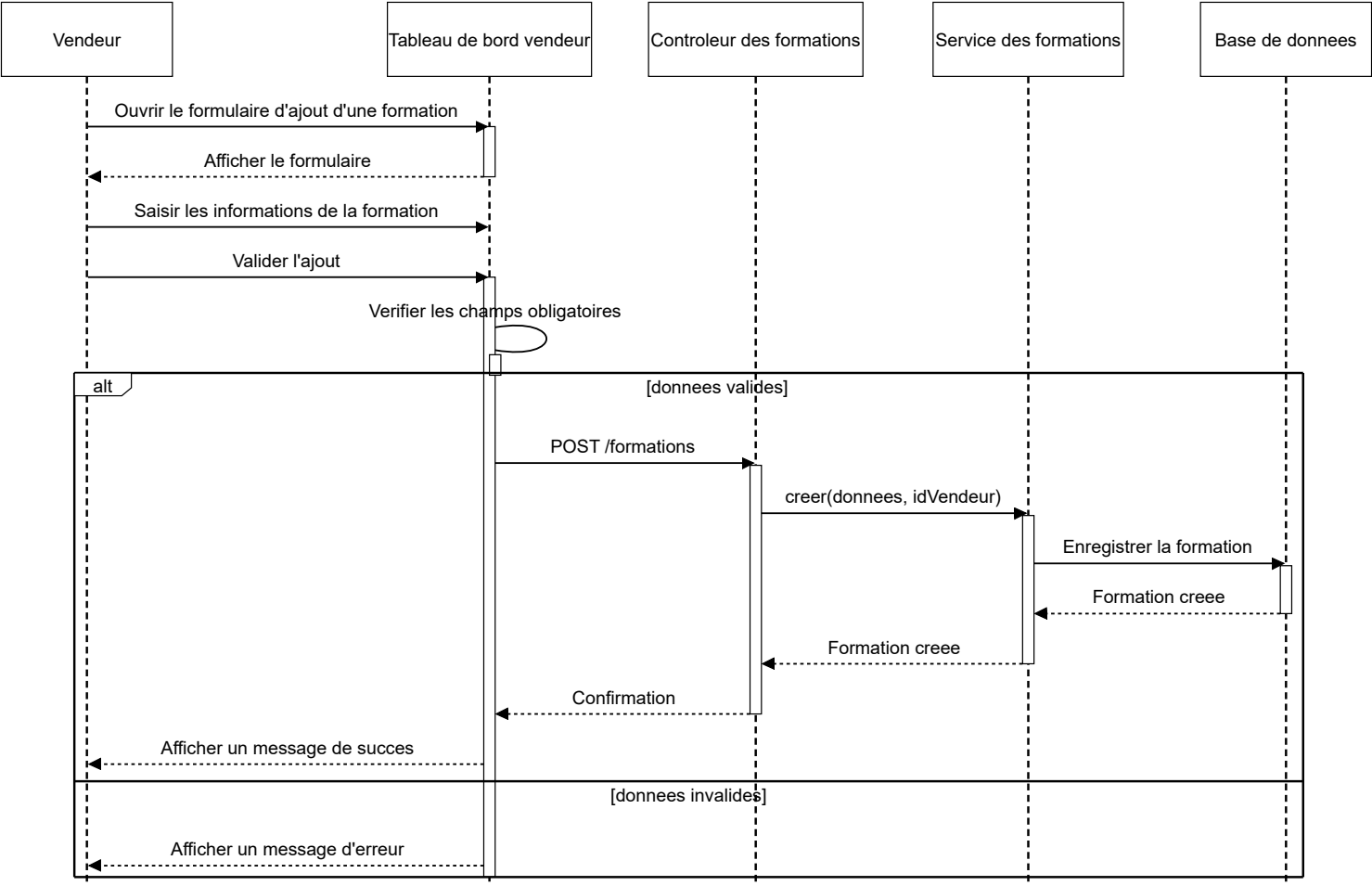
Diagramme de sequence - Ajout d'une formation
