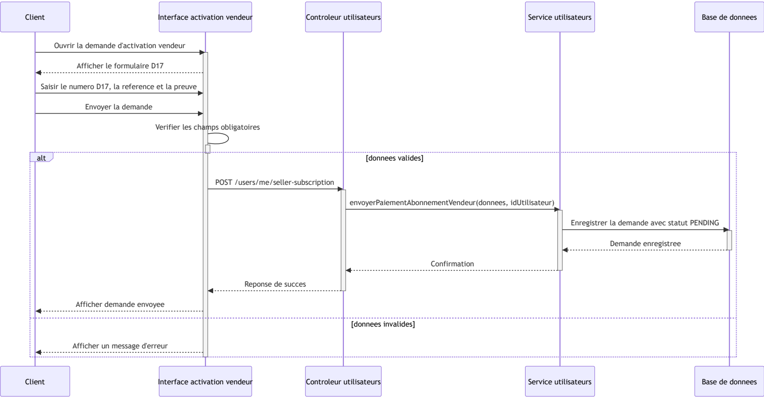
Diagramme de séquence - Demande d'activation vendeur
