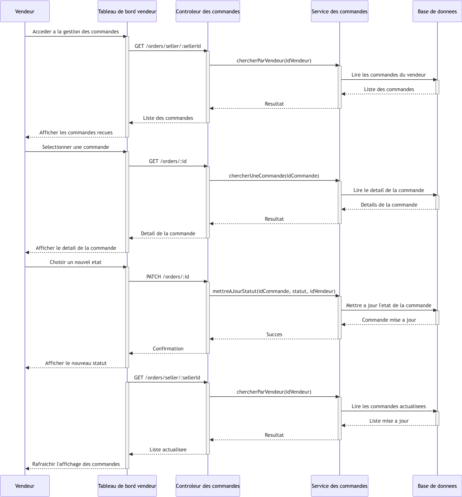
Diagramme de séquence - Gestion des commandes vendeur
