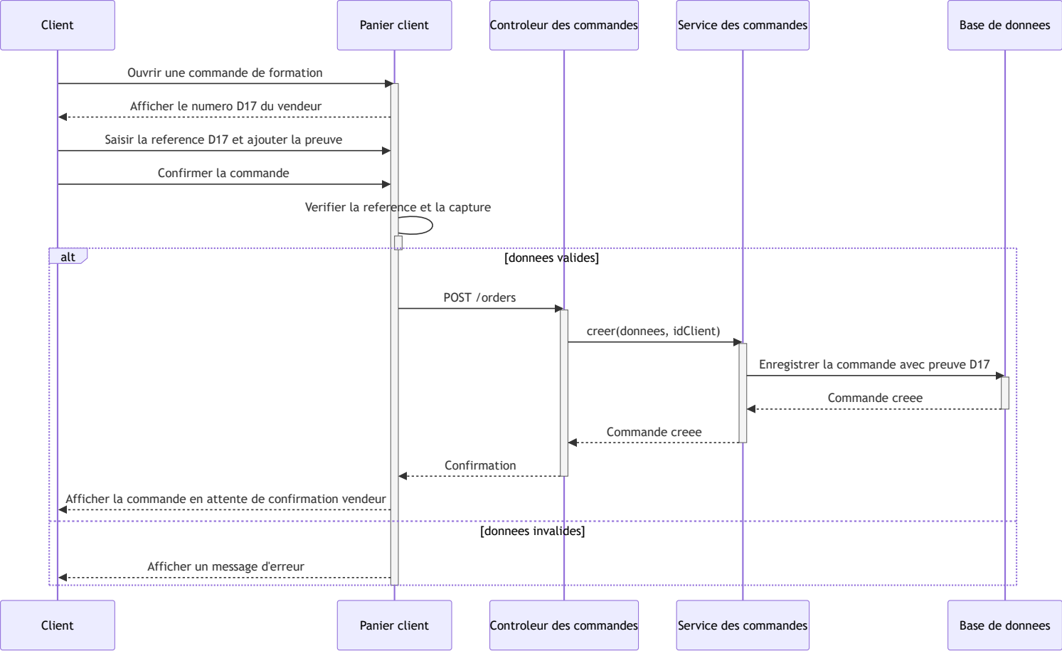
Diagramme de séquence - Paiement D17 client
