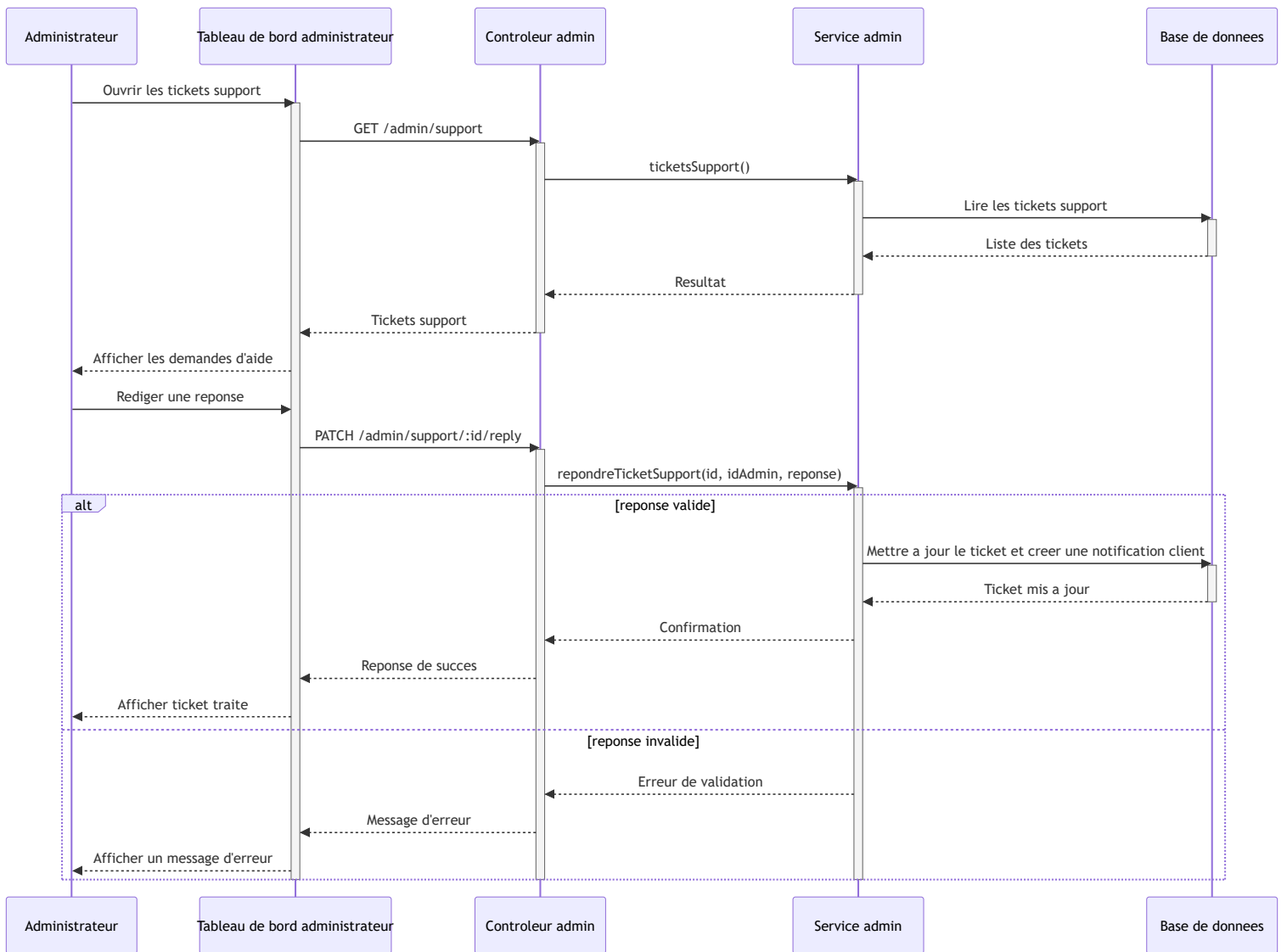
Diagramme de séquence - Traitement d'un ticket support
