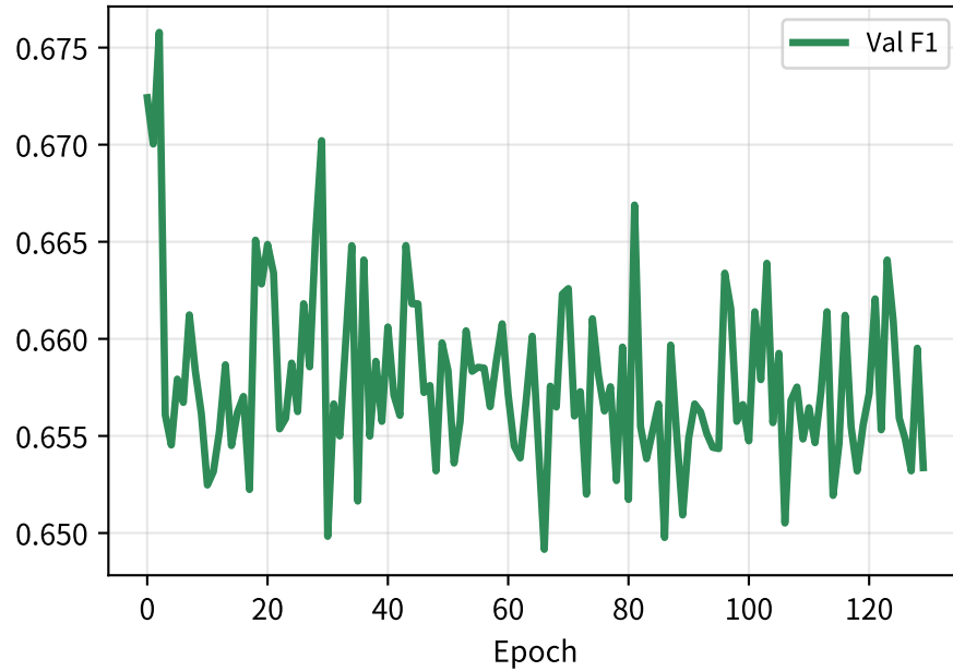
F1 Score
