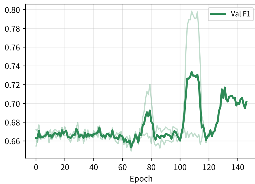
F1 Score
