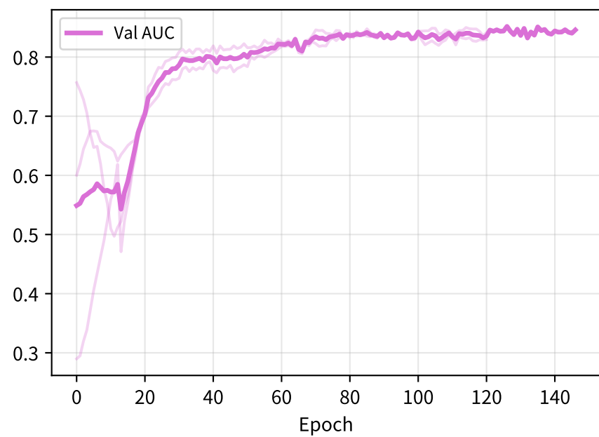
AUC-ROC
