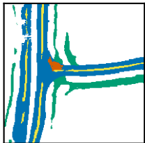
Mittelwert ( z = \mu )
