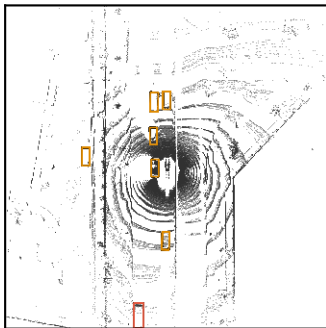
Weltmodell (Vorhersage)
