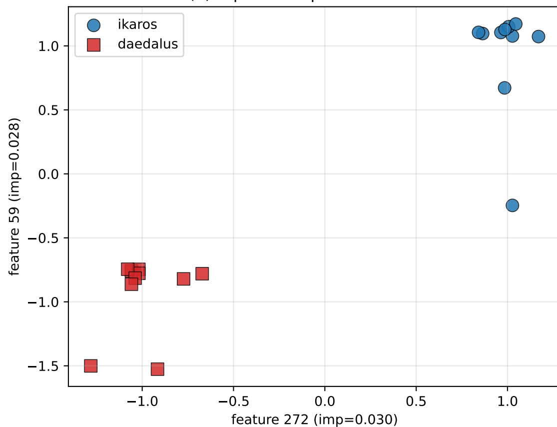
(d) Top-2 RF-important features
