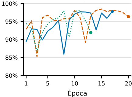
CNN compacta
