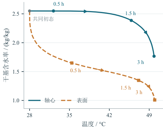
(a) 温湿状态路径
