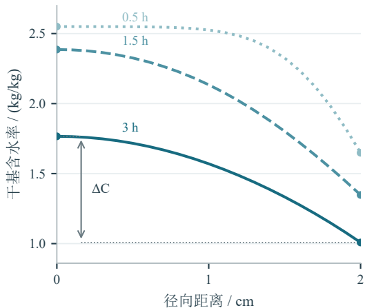
(b) 含水率径向剖面
