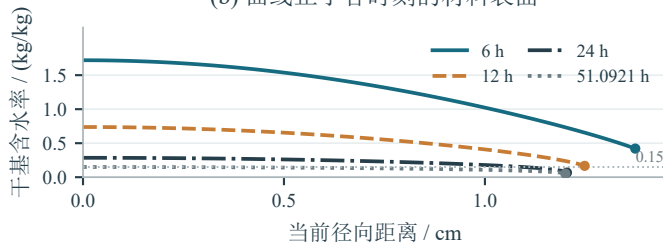
(b) 曲线止于各时刻的材料表面
