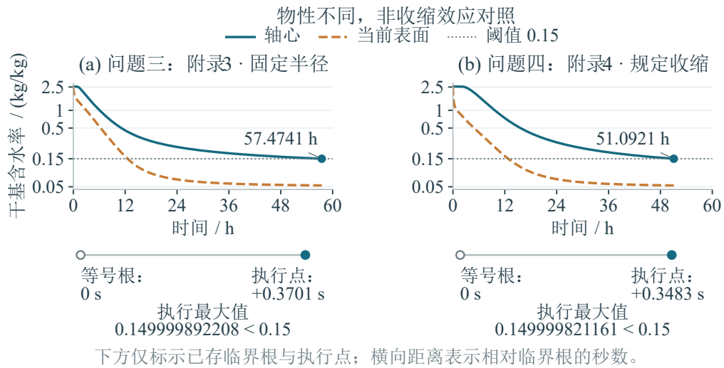
图 8 问题三(左)与问题四(右)的干燥过程与事件判定。上排为一维径向有效模型的轴心、当前表面含水率演化。纵轴为对数刻度，水平线为 0.15 kg/kg 阈值，终点标记对应各自正式执行时刻。下排以各自临界根为时间原点，仅标示已存临界根与执行点，并列出行执行最大值。两问采用各自附录物性，问题四另施加观测半径历程，因而曲线差异不能全部归因于收缩。
