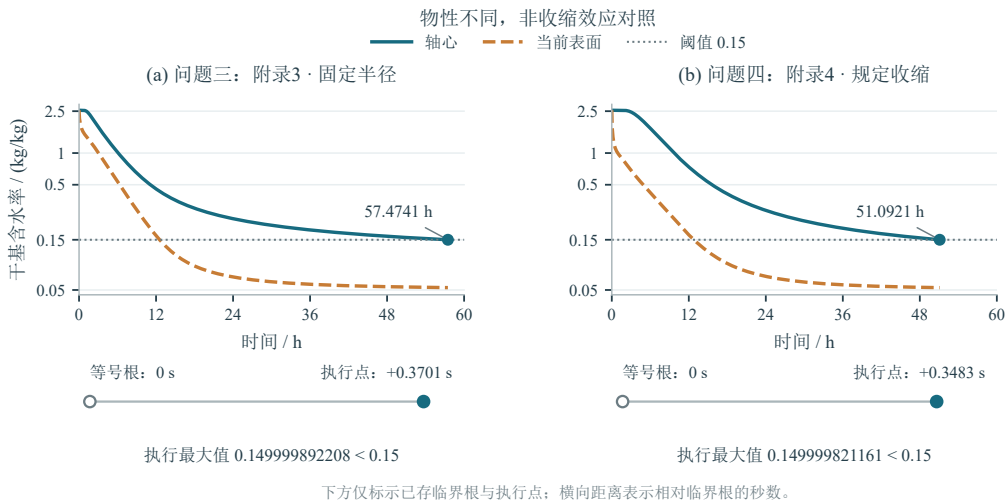
图 8 问题三（左）与问题四（右）的干燥过程与事件判定。上排为一维径向有效模型的轴心、当前表面含水率演化。纵轴为对数刻度，水平线为 0.15 kg/kg 阈值，终点标记对应各自正式执行时刻。下排以各自临界根为时间原点，仅标示已存临界根与执行点，并列出执行最大值。两问采用各自附录物性，问题四另施加观测半径历程，因而曲线差异不能全部归因于收缩。
