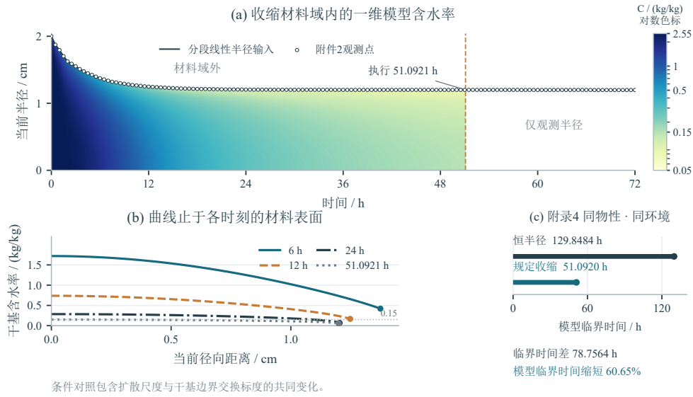
图 10 规定收缩下的径向有效模型场、观测输入与同物性条件对照。(a) 当前实际半径坐标中的含水率色图仅显示至正式执行时刻，采用对数色标；全部观测点及分段线性半径输入保留至 72h，执行线之后只展示半径。(b) 各时刻含水率剖面止于当时材料表面。(c) 附录 4 同物性、同环境下的恒半径与规定收缩临界根对照。临界根与执行时刻分别标示；时间差包含扩散尺度和干基边界交换标度变化。
