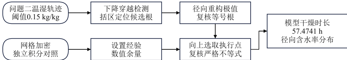
图 7 问题三的一维径向终点判定流程
