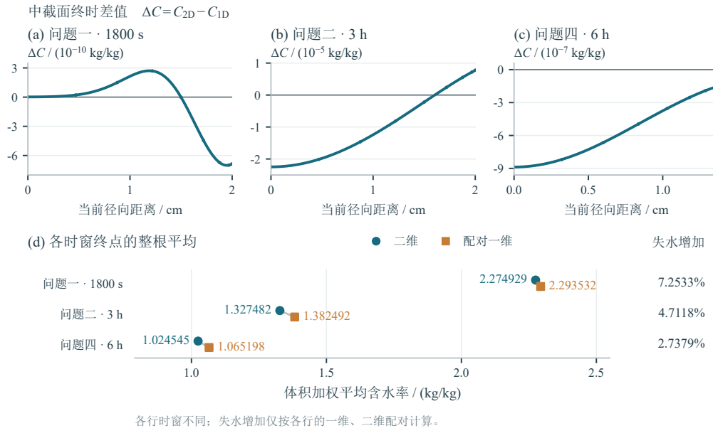
图 11 已保存一维、二维配对场的降维证据：上排为问题一 1800 s、问题二 10800 s 及问题四 21600 s 的中截面径向含水率差 \Delta C = C_{2D} - C_{1D} ；下排为各时窗终点的整根体积加权平均，圆点、方点分别表示二维和配对一维，终点失水增加与表7一致。问题一、二在已检时段中截面采样最大含水率差分别为 4.09 \times 10^{-9} 、 2.24706 \times 10^{-5} \text{ kg/kg} 。上述时段最大差与上排终点差值的统计范围不同。体积加权平均在空间均匀干密度假设下等于干质量加权平均。数据取自同网格一维、二维配对保存场，文件索引与哈希见支撑材料图表来源清单；二维半柱坐标的 z = 0 为中截面对称面。
