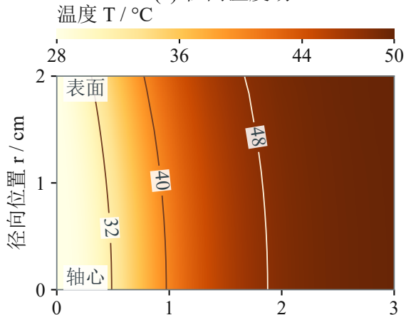
(a) 径向温度场
