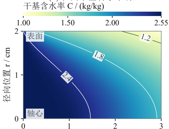
(b) 径向干基含水率场
