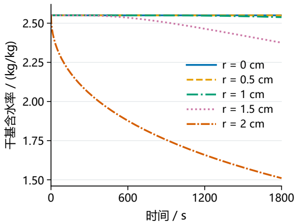
(b) 干基含水率随时间变化
