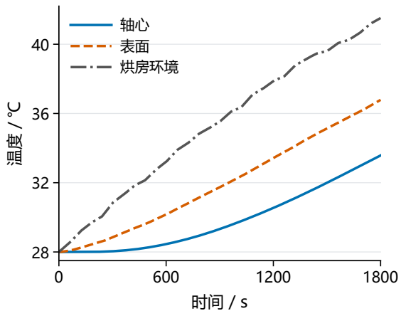
(a) 温度随时间变化
