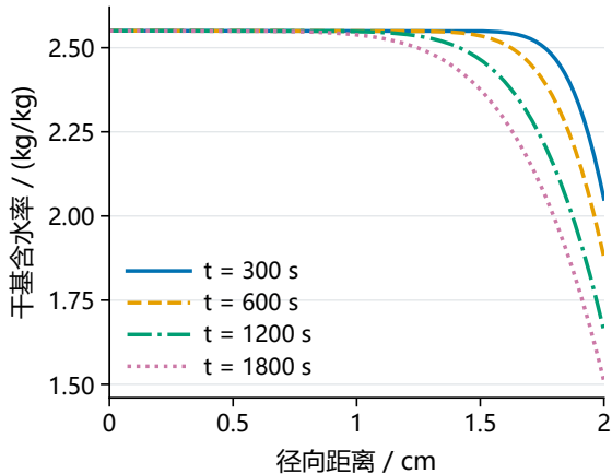
(b) 干基含水率径向分布
