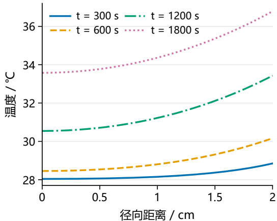
(a) 温度径向分布
