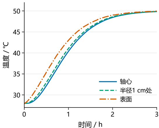
(a) 温度随时间变化
