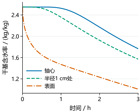
(b) 干基含水率随时间变化
