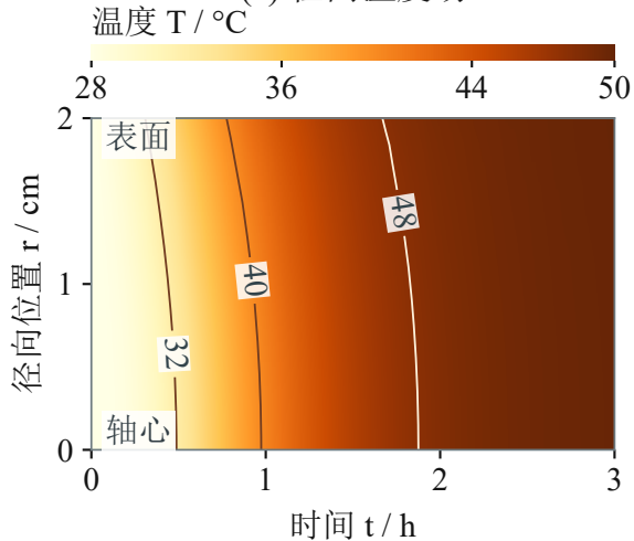
(a) 径向温度场
