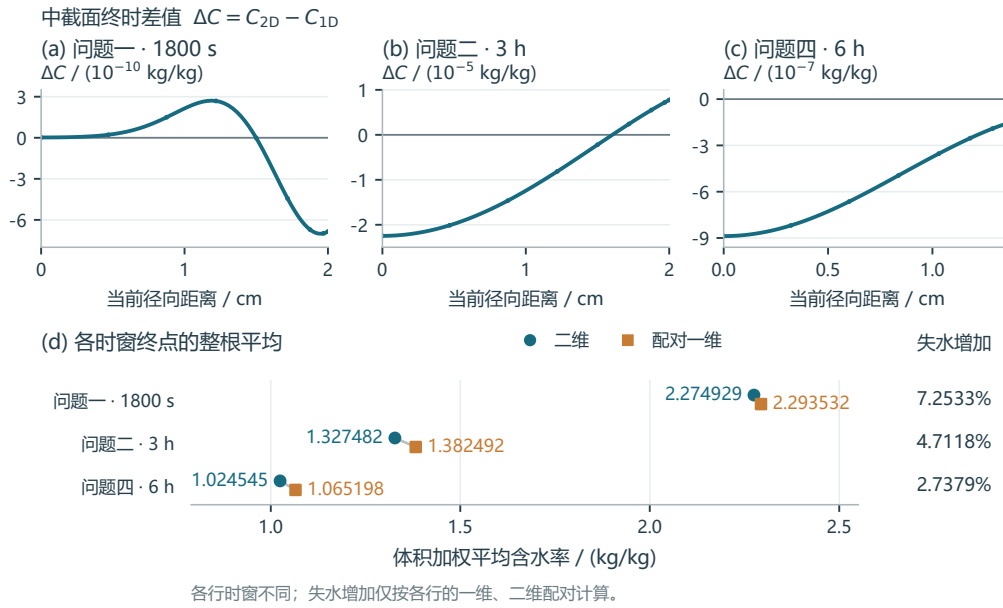
图 6 已保存一维、二维配对场的降维证据：上排为问题一 1800s、问题二 10800s 及问题四 21600s 的中截面径向含水率差 \Delta C = C_{2D} - C_{1D} ；下排为各时窗终点的整根体积加权平均，圆点、方点分别表示二维和配对一维，终点失水增加与表7一致。问题一、二在已检时段中截面采样最大含水率差分别为 4.09 \times 10^{-9} 、 2.24706 \times 10^{-5} \text{ kg/kg} 。上述时段最大差与上排终点差值的统计范围不同。体积加权平均在空间均匀干密度假设下等于干质量加权平均。数据取自同网格一维、二维配对保存场，文件索引与哈希见支撑材料图表来源清单；二维半柱坐标的 z = 0 为中截面对称面。
