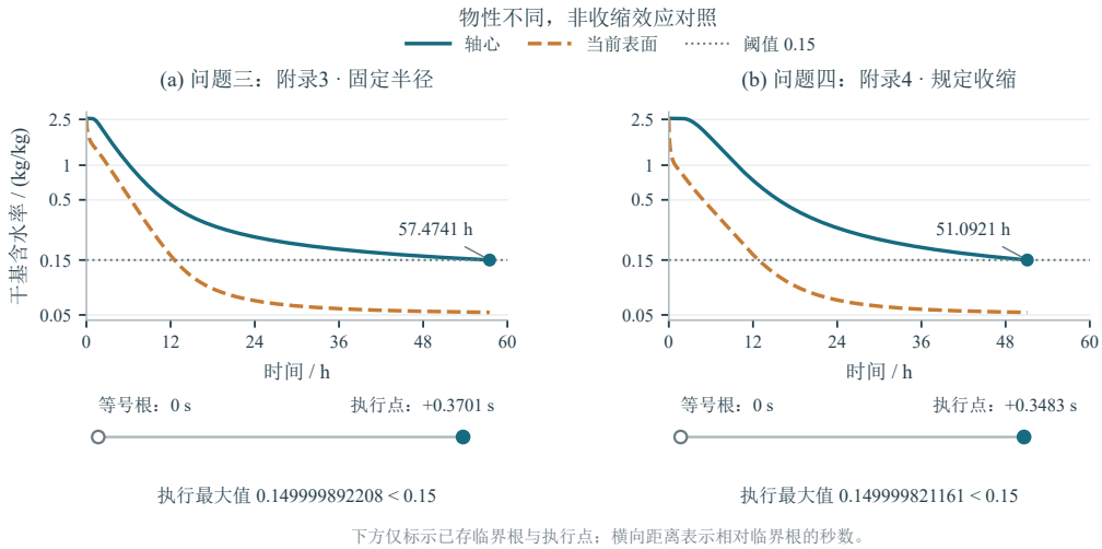
图 6 问题三（左）与问题四（右）的干燥过程与事件判定。上排为一维径向有效模型的轴心、当前表面含水率演化。纵轴为对数刻度，水平线为 0.15 kg/kg 阈值，终点标记对应各自正式执行时刻。下排以各自临界根为时间原点，仅标示已存临界根与执行点，并列出执行最大值。两问采用各自附录物性，问题四另施加观测半径历程，因而曲线差异不能全部归因于收缩。
