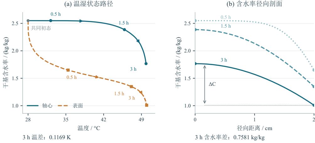
图 5 第二问前 3 小时的温湿状态路径与径向含水率。左图连接轴心和表面的已存温湿状态，箭头表示时间推进；右图保留中截面径向剖面，双向箭头标示末时轴心与表面含水率差。
