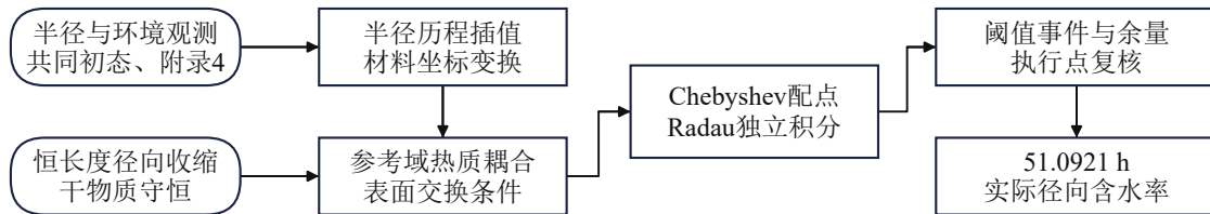
图 8 问题四的收缩模型求解流程
