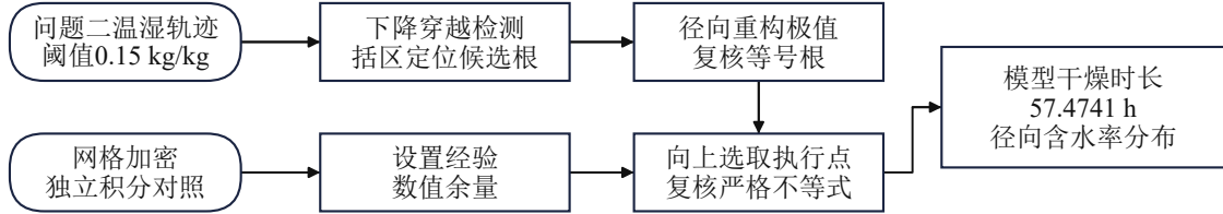
图 6 问题三的一维径向终点判定流程
