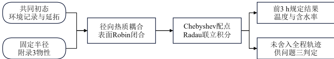
图 4 问题二求解流程
