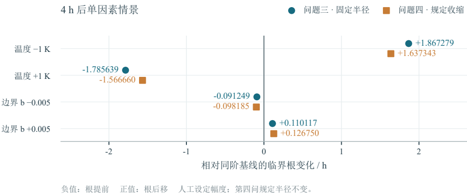
图 11 后段环境情景相对同阶基线的根变化：幅度为人工设定，第四问规定半径保持不变。圆点、方点分别表示问题三、四，共用零线；负值表示根提前，正值表示根后移。
