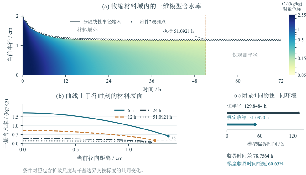
图 9 规定收缩下的径向有效模型场、观测输入与同物性条件对照。(a) 当前实际半径坐标中的含水率色图仅显示至正式执行时刻，采用对数色标；全部观测点及分段线性半径输入保留至 72 h，执行线之后只展示半径。(b) 各时刻含水率剖面止于当时材料表面。(c) 附录 4 同物性、同环境下的恒半径与规定收缩临界根对照。临界根与执行时刻分别标示；时间差包含扩散尺度和干基边界交换标度变化。
