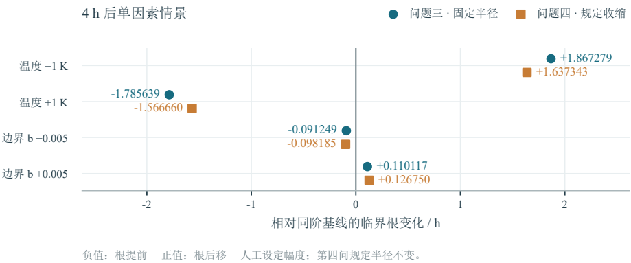
图 11 后段环境情景相对同阶基线的根变化：幅度为人工设定，第四问规定半径保持不变。圆点、方点分别表示问题三、四，共用零线；负值表示根提前，正值表示根后移。
