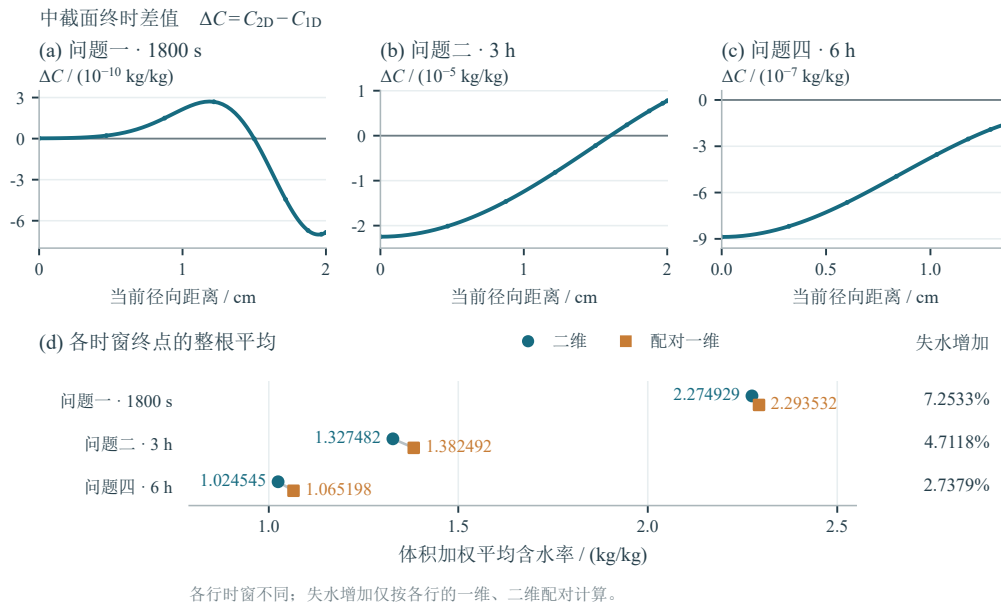
图 10 已保存一维、二维配对场的降维证据：上排为问题一 1800 s、问题二 10800 s 及问题四 21600 s 的中截面径向含水率差 \Delta C = C_{2D} - C_{1D} ；下排为各时窗终点的整根体积加权平均，圆点、方点分别表示二维和配对一维，终点失水增加与表7一致。问题一、二在已检时段中截面采样最大含水率差分别为 4.09 \times 10^{-9} 、 2.24706 \times 10^{-5} \text{ kg/kg} 。上述时段最大差与上排终点差值的统计范围不同。体积加权平均在空间均匀干密度假设下等于干质量加权平均。数据取自同网格一维、二维配对保存场，文件索引与哈希见支撑材料图表来源清单；二维半柱坐标的 z = 0 为中截面对称面。
