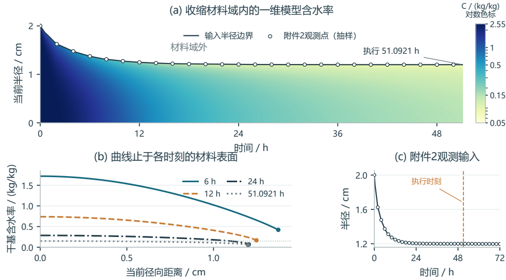
图 4 规定收缩下的径向有效模型场与观测输入。(a) 当前实际半径坐标中的含水率色图，仅显示至正式执行时刻，采用对数色标，材料域外留白；边界线与空心点区分输入半径及抽样观测记录。(b) 附录 4 下不同时间的径向含水率剖面。(c) 完整观测半径历程。半径图标出正式执行时刻；剖面采用当前实际半径坐标，各曲线只画至对应时刻的材料表面。
