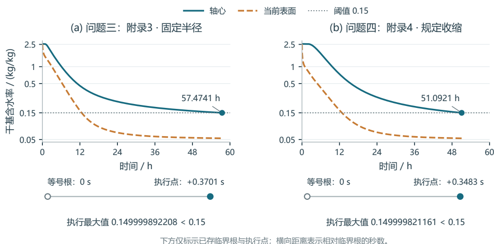
图 3 问题三（左）与问题四（右）的干燥过程与事件判定。上排为一维径向有效模型的轴心、当前表面含水率演化。纵轴为对数刻度，水平线为 0.15 kg/kg 阈值，终点标记对应各自正式执行时刻。下排以各自临界根为时间原点，仅标示已存临界根与执行点，并列出执行最大值。两问采用各自附录物性，问题四另施加观测半径历程，因而曲线差异不能全部归因于收缩。
