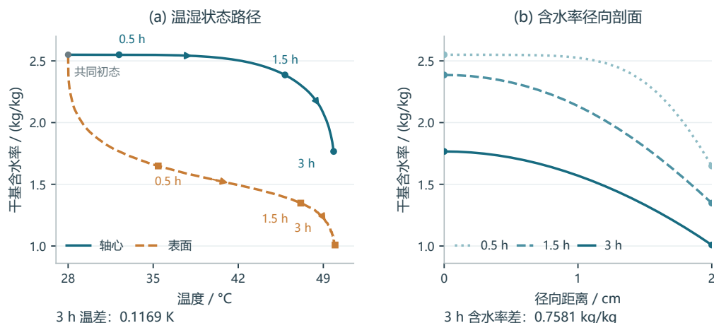
图 2 第二问前 3 小时的温湿状态路径与径向含水率。左图以温度、干基含水率为坐标，分别连接轴心和表面的已保存状态，箭头表示时间推进；右图保留对应时刻的中截面径向剖面。
