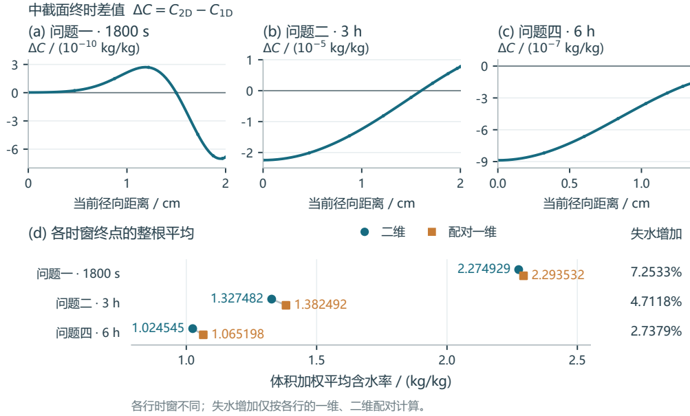
图 5 已保存一维、二维配对场的降维证据：上排为问题一 1800 s、问题二 10800 s 及问题四 21600 s 的中截面径向含水率差 \Delta C = C_{2D} - C_{1D} ；下排为各时窗终点的整根体积加权平均，圆点、方点分别表示二维和配对一维，终点失水增加与表7一致。问题一、二在已检时段中截面采样最大含水率差分别为 4.09 \times 10^{-9} 、 2.24706 \times 10^{-5} kg/kg。上述时段最大差与上排终点差值的统计范围不同。体积加权平均在空间均匀干密度假设下等于干质量加权平均。来源：q4_complete_delivery/v1/validation/geometry/ 下的 q1_80x128/q1_80x0、q2_3_80x256_integral/q23_80x0_integral 及 q4_80x128_integral/q4_80x0_integral 配对.npz 文件；二维半柱坐标的 z = 0 为中截面对称面。
