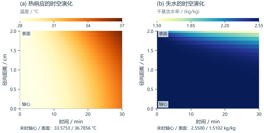
图 1 第一问的时间-径向温湿场。横轴为时间，纵轴为径向距离；左、右色标分别表示温度与干基含水率，均由已保存采样值着色。
