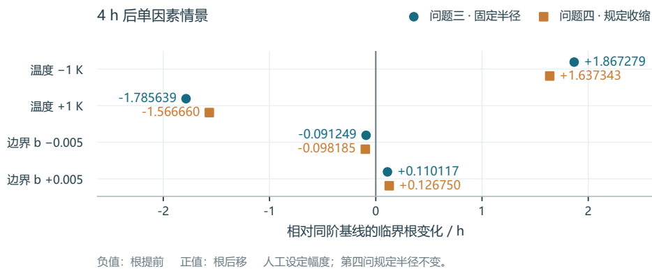
图 6 后段环境情景相对同阶基线的根变化；幅度为人工设定，第四问规定半径保持不变。圆点、方点分别表示问题三、四，共用零线；负值表示根提前，正值表示根后移。
