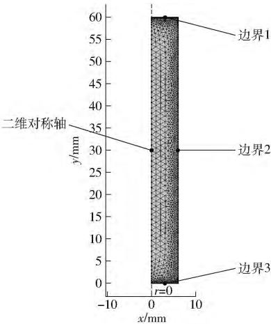
图4 二维轴对称模型及边界名称
