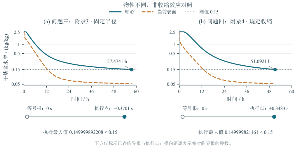
图 4 问题三（左）与问题四（右）的干燥过程与事件判定。上排为一维径向有效模型的轴心、当前表面含水率演化。纵轴为对数刻度，水平线为 0.15 kg/kg 阈值，终点标记对应各自正式执行时刻。下排以各自临界根为时间原点，仅标示已存临界根与执行点，并列出执行最大值。两问采用各自附录物性，问题四另施加观测半径历程，因而曲线差异不能全部归因于收缩。
