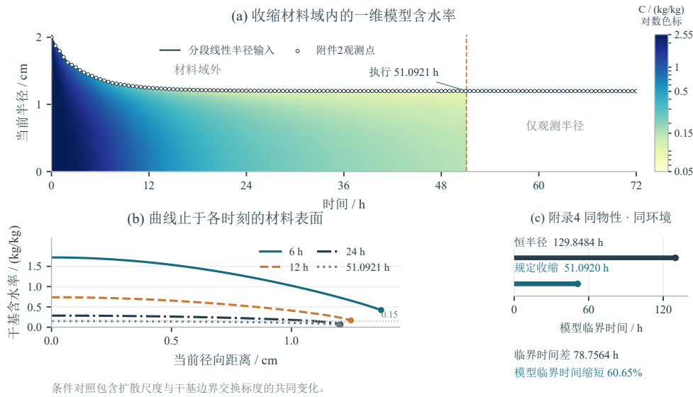
图 5 规定收缩下的径向有效模型场、观测输入与同物性条件对照。(a) 当前实际半径坐标中的含水率色图仅显示至正式执行时刻，采用对数色标；全部观测点及分段线性半径输入保留至 72h，执行线之后只展示半径。(b) 各时刻含水率剖面止于当时材料表面。(c) 附录 4 同物性、同环境下的恒半径与规定收缩临界根对照。临界根与执行时刻分别标示；时间差包含扩散尺度和干基边界交换标度变化。
