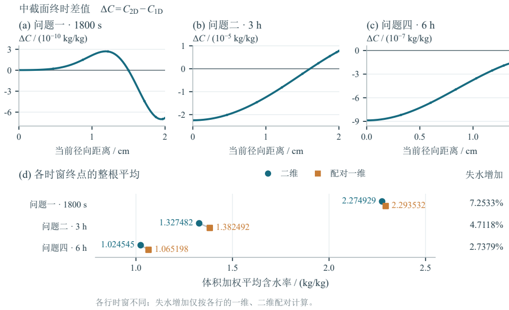
图 6 已保存一维、二维配对场的降维证据：上排为问题一 1800 s、问题二 10800 s 及问题四 21600 s 的中截面径向含水率差 \Delta C = C_{2D} - C_{1D} ；下排为各时窗终点的整根体积加权平均，圆点、方点分别表示二维和配对一维，终点失水增加与表7一致。问题一、二在已检时段中截面采样最大含水率差分别为 4.09 \times 10^{-9} 、 2.24706 \times 10^{-5} \text{ kg/kg} 。上述时段最大差与上排终点差值的统计范围不同。体积加权平均在空间均匀干密度假设下等于干质量加权平均。数据取自同网格一维、二维配对保存场，文件索引与哈希见支撑材料图表来源清单；二维半柱坐标的 z = 0 为中截面对称面。
