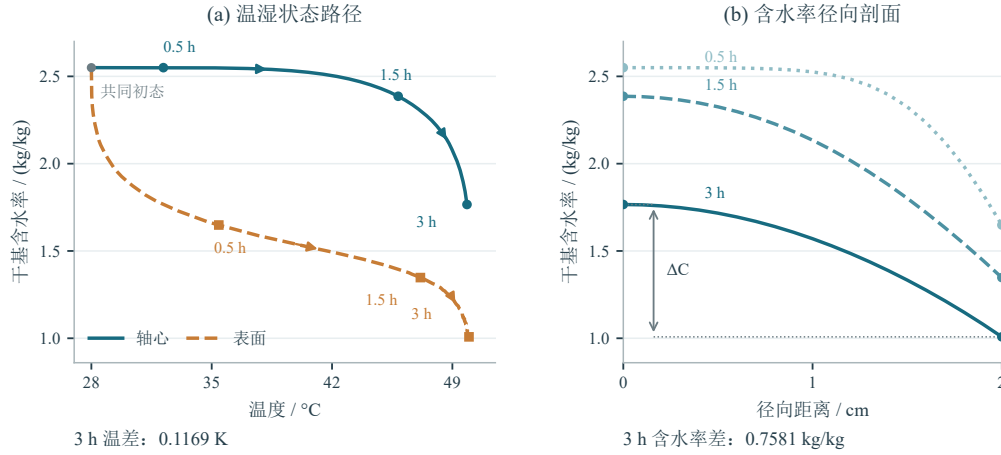
图 3 第二问前 3 小时的温湿状态路径与径向含水率。左图连接轴心和表面的已存温湿状态，箭头表示时间推进；右图保留中截面径向剖面，双向箭头标示末时轴心与表面含水率差。
