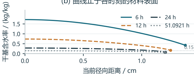
(b) 曲线止于各时刻的材料表面
