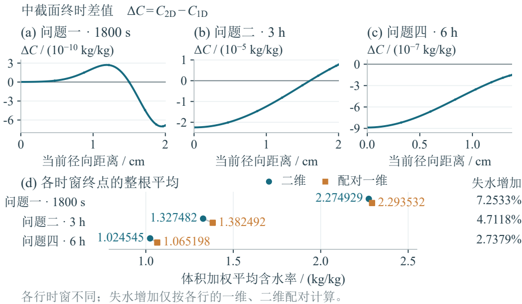
图 11 已保存一维、二维配对场的降维证据：上排为问题一 1800 s、问题二 10800 s 及问题四 21600 s 的中截面径向含水率差 \Delta C = C_{2D} - C_{1D} ；下排为各时窗终点的整根体积加权平均，圆点、方点分别表示二维和配对一维，终点失水增加与表7一致。问题一、二在已检时段中截面采样最大含水率差分别为 4.09 \times 10^{-9} 、 2.24706 \times 10^{-5} \text{ kg/kg} 。上述时段最大差与上排终点差值的统计范围不同。体积加权平均在空间均匀干密度假设下等于干质量加权平均。数据取自同网格一维、二维配对保存场，文件索引与哈希见支撑材料图表来源清单；二维半柱坐标的 z = 0 为中截面对称面。
